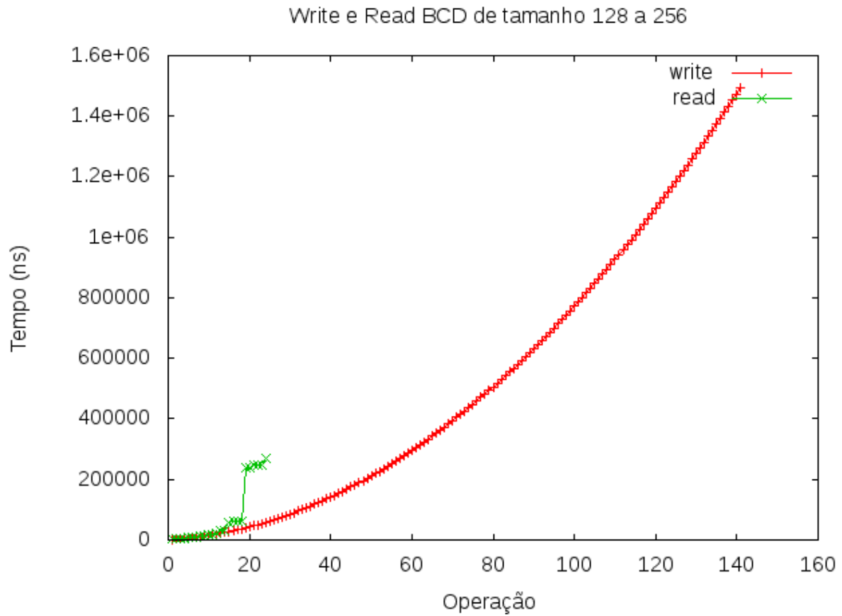
Figura 5.11: Buffer com fila de tamanho 128 à 256.
