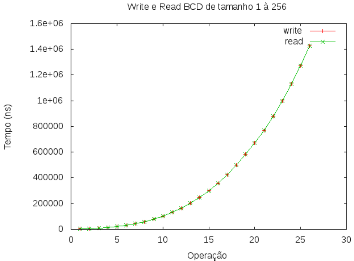
Figura 5.13: Buffer com fila de tamanho 1 a 256.
