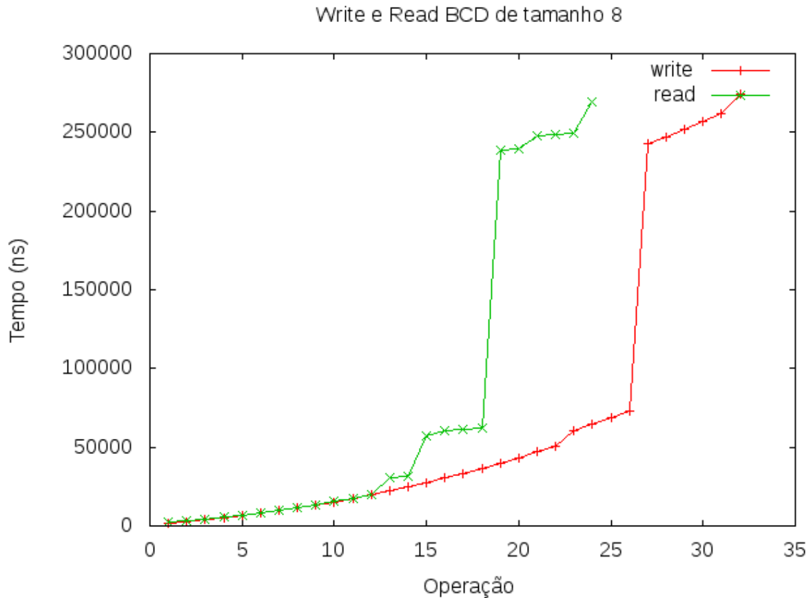
Figura 5.7: Buffer com fila de tamanho 8.
