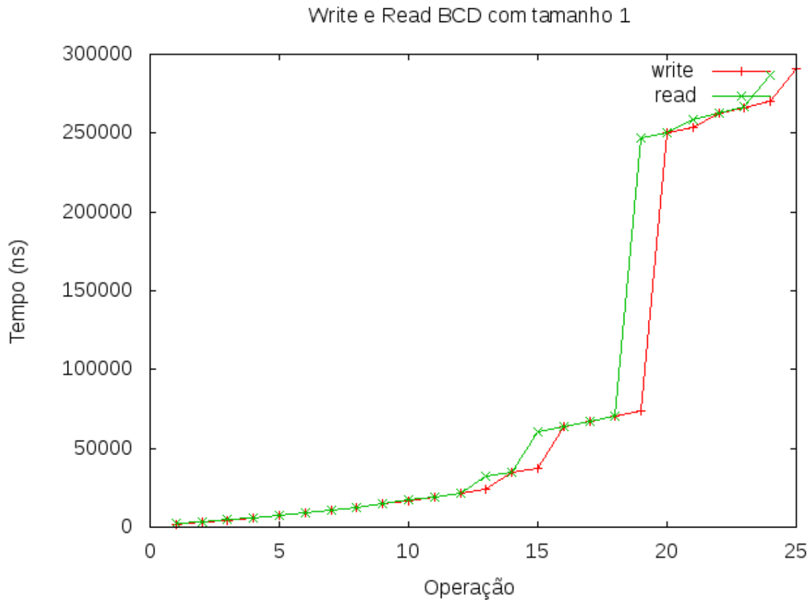
Figura 5.4: Buffer com fila de tamanho 1.
