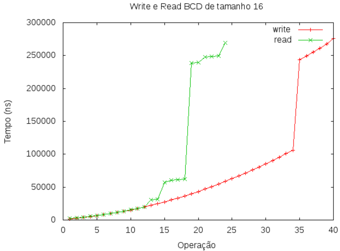
Figura 5.8: Buffer com fila de tamanho 16.
