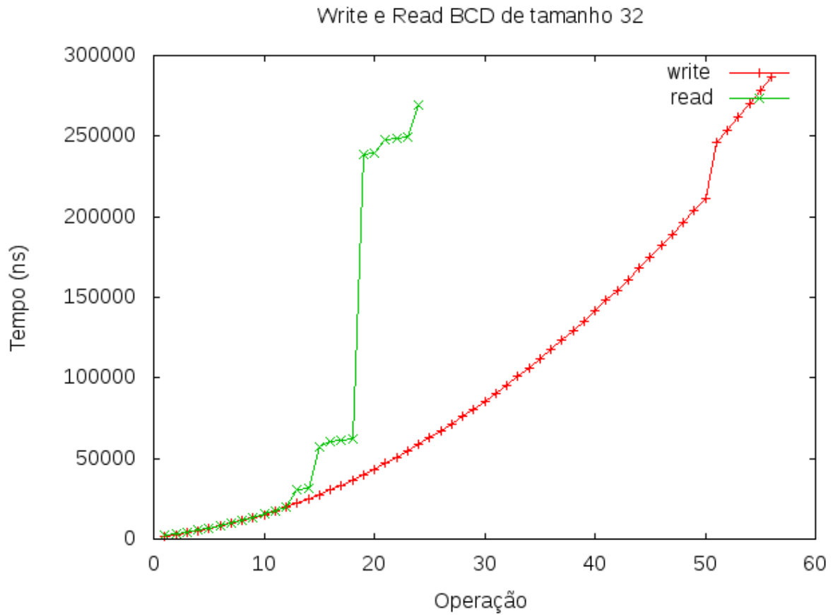
Figura 5.9: Buffer com fila de tamanho 32.
