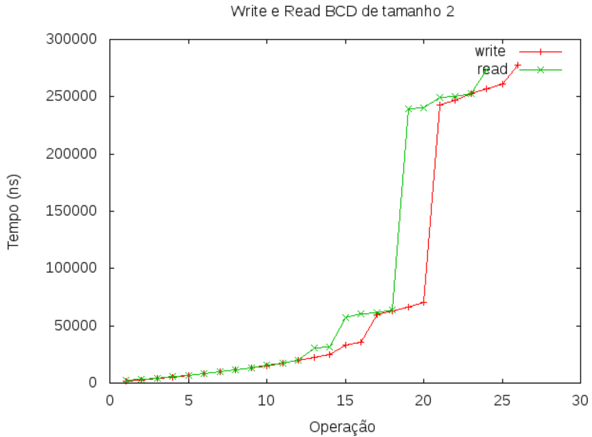
Figura 5.5: Buffer com fila de tamanho 2.
