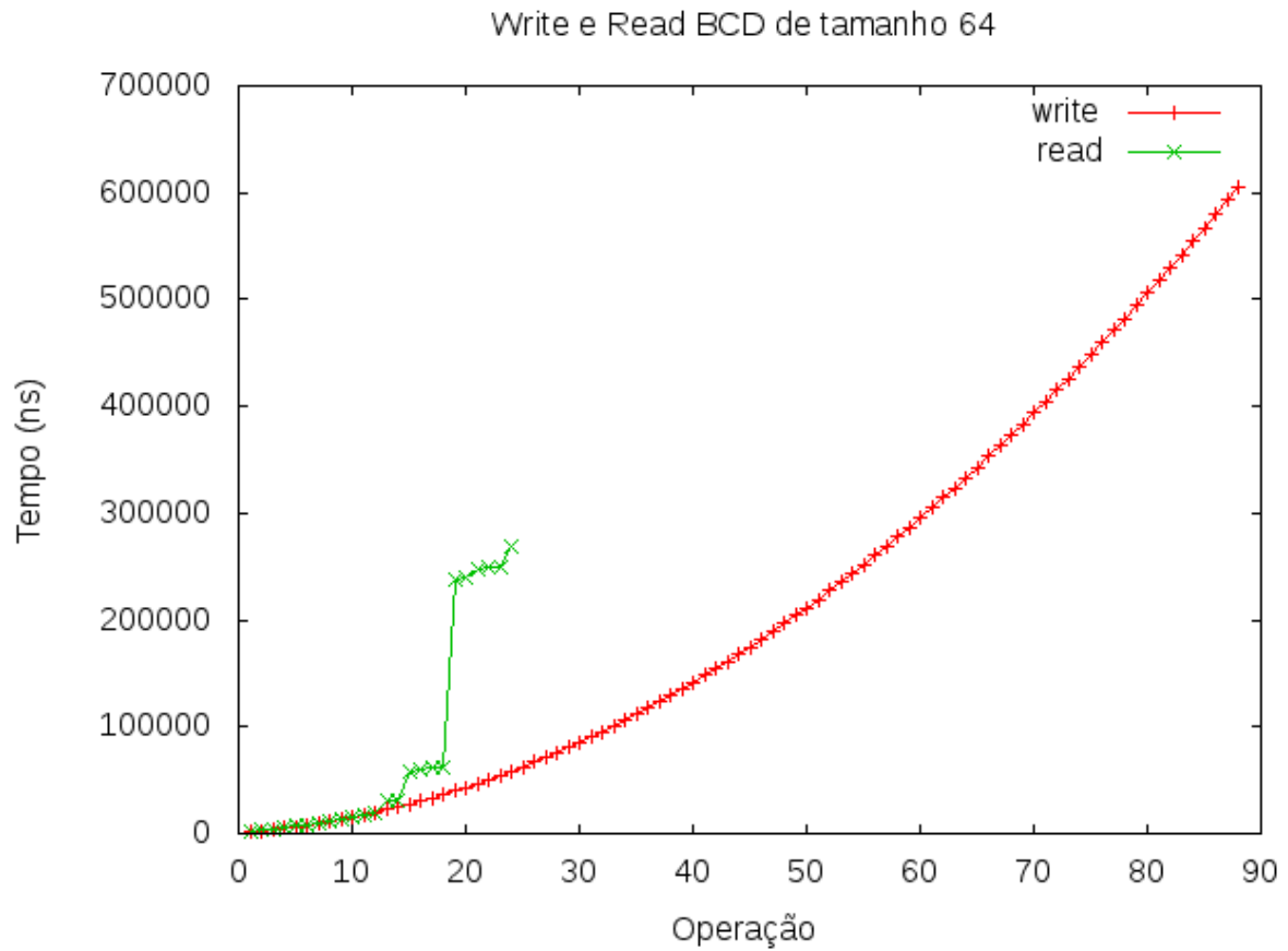
Figura 5.10: Buffer com fila de tamanho 64.
