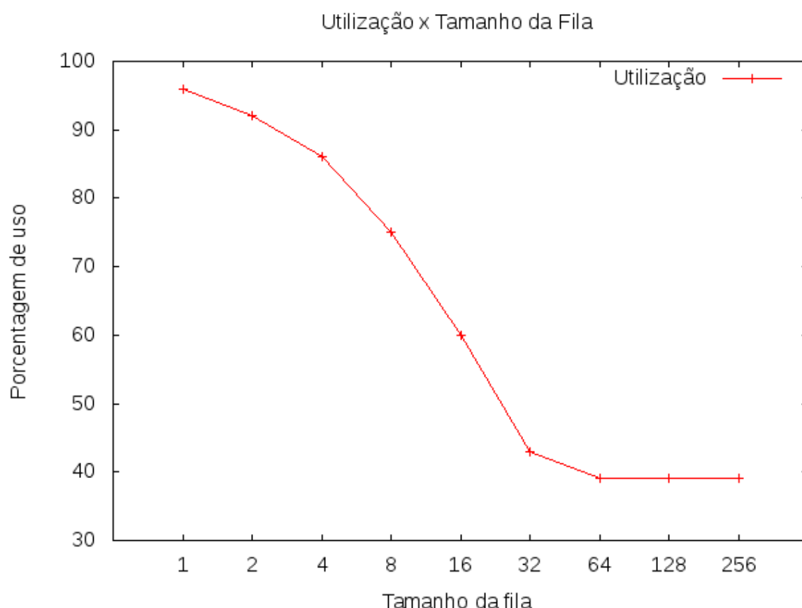
Figura 5.12: Uso do Buffer em porcentagem em relação com o tamanho da fila.
