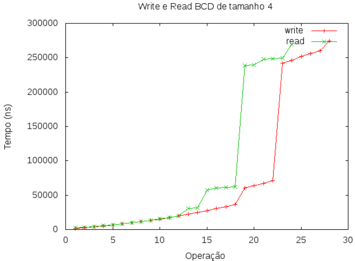
Figura 5.6: Buffer com fila de tamanho 4.
